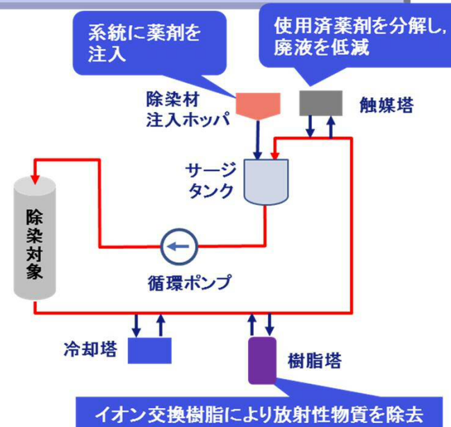
系統除染の例(化学的除染の場合)
