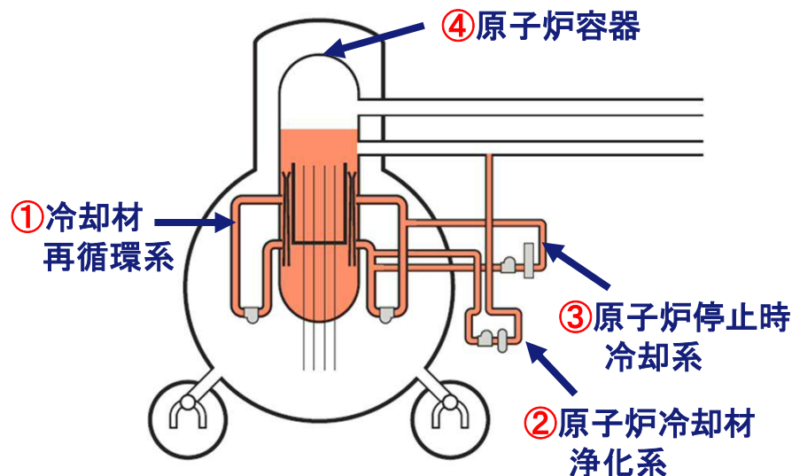
系統除染の範囲(想定)
