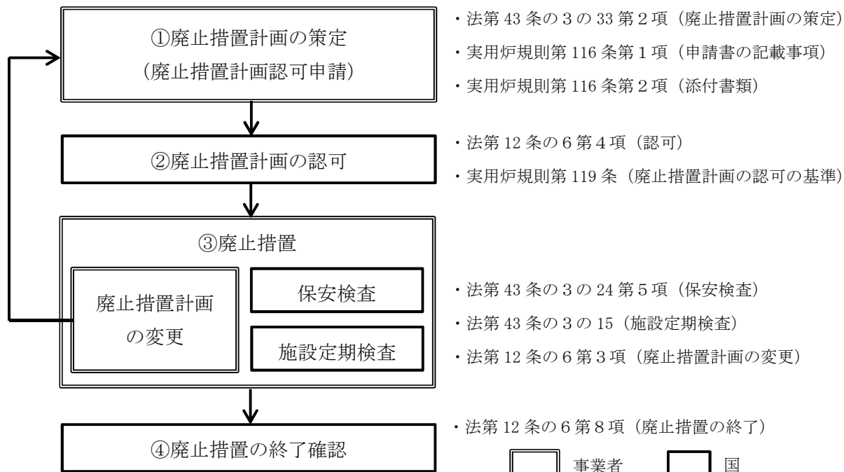
廃止措置の流れと関連法令との関係
