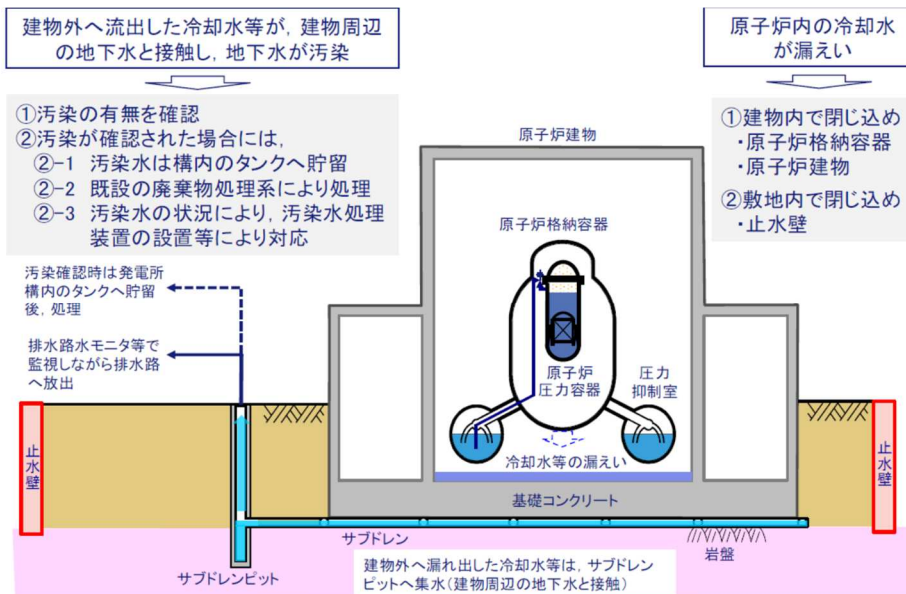
図5-31 汚染水の外部流出防止対策
