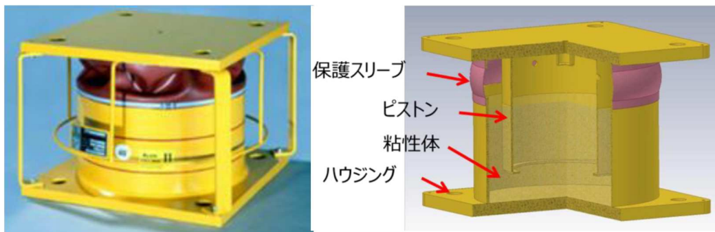
図5-2 制震装置の外観及び構造
