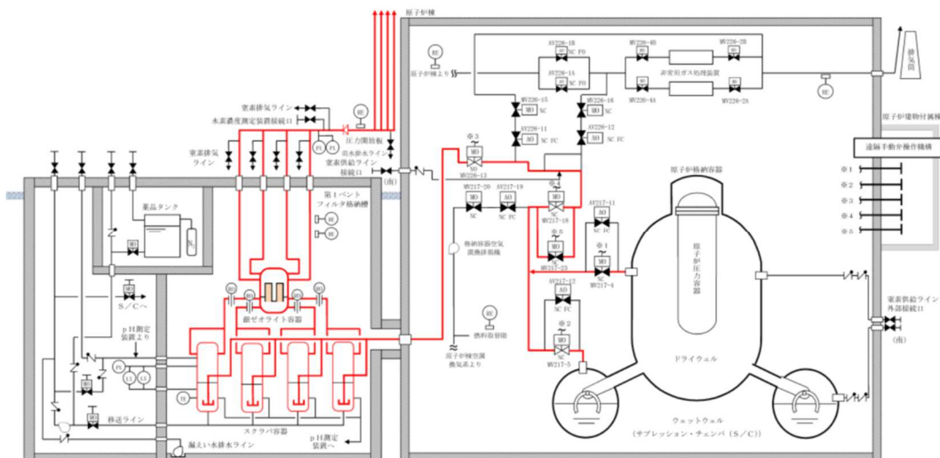
図 5-23 格納容器フィルタベント系
