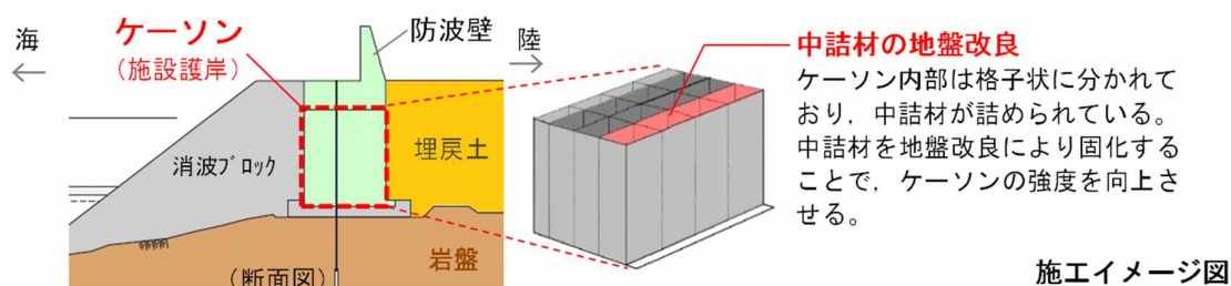
図5-6 ケーソンの耐震補強（イメージ）
