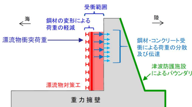
図5-8 漂流物対策工（イメージ）
