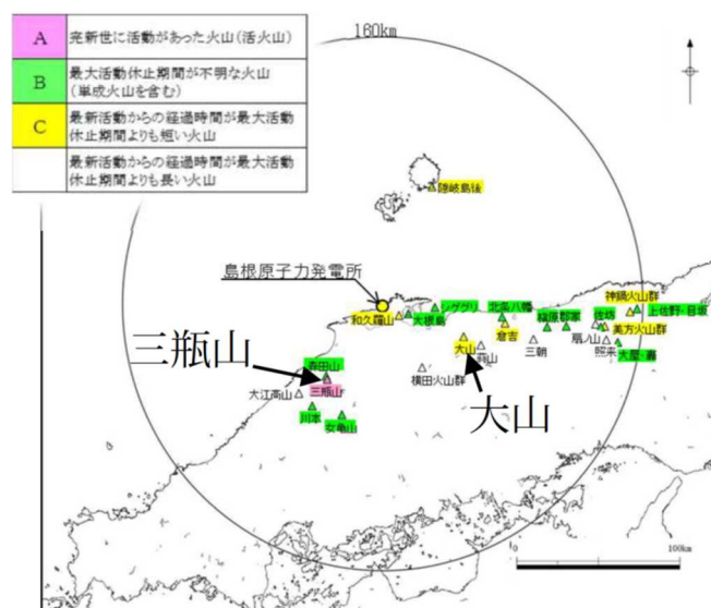
図5-9 発電所周辺の火山
