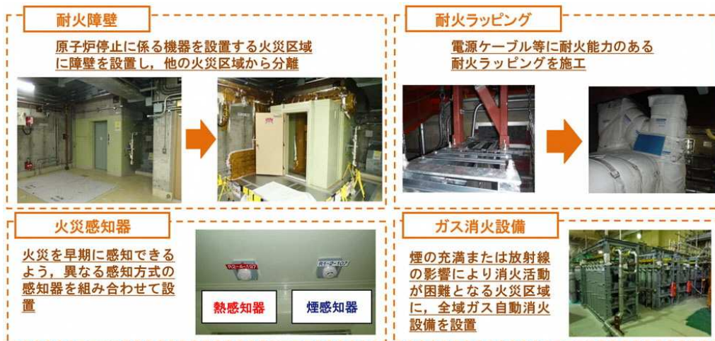
図 5-1-4 火災防護対策の例
