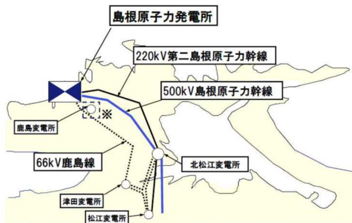
図5-16 発電所への送電系統
