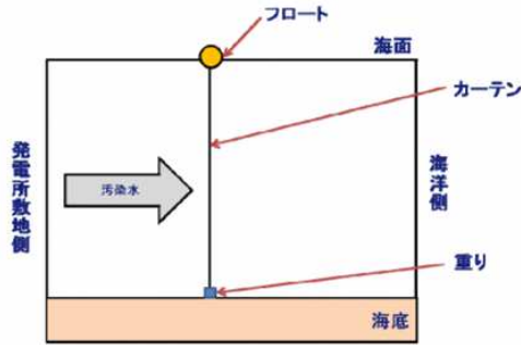
図5-29 シルトフェンスの概念図
