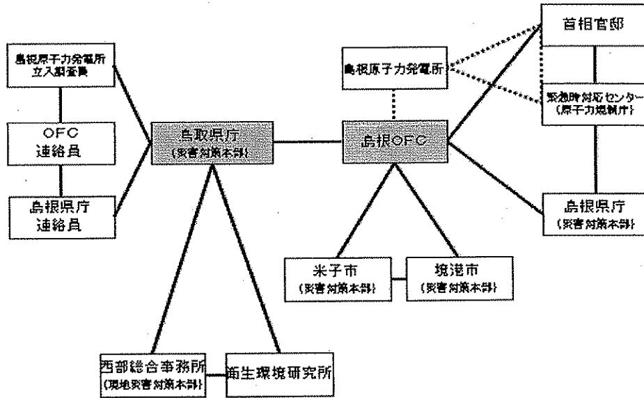
(イ) 原子力防災ネットワーク図
